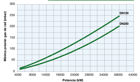
HTLX3050 PR-MD con válvulas neumáticas
