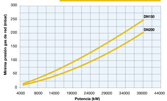
TLX3050 PR-MD con válvulas neumáticas
